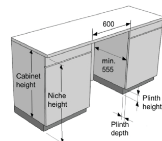
Niche dimensions
